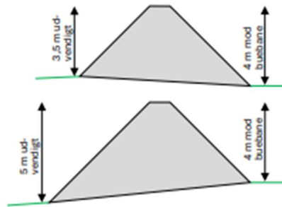
Anlæg i terræn, øverst mod nordøst, nederst mod vest og nordvest i 1/200
