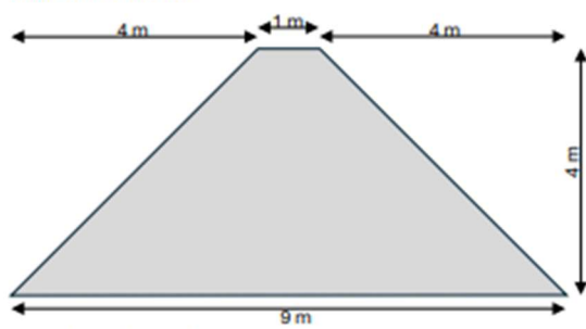
Principprofil af sikkerhedsvolde i 1/100
